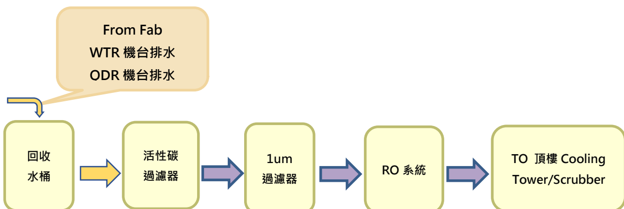
圖 41_辛耘公司廠房製程一般酸廢水回收流程
